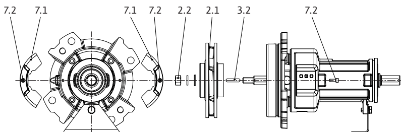
Fig. 29: A betolható egység összeszerelése
