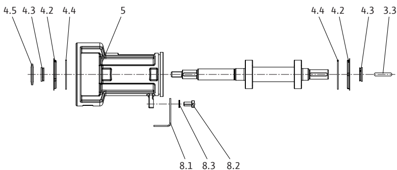
Fig. 23: Csapágybak
