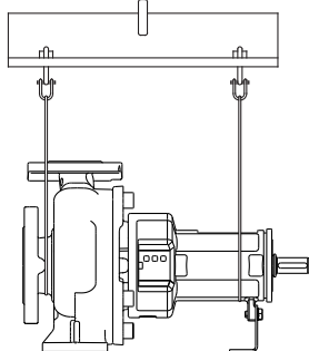
Fig. 3: Szivattyú rögzítése
