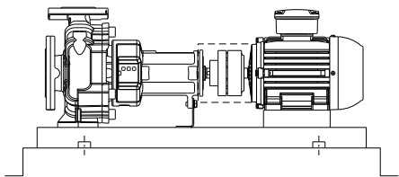
Fig. 5: A gépcsoport alapra szerelése
