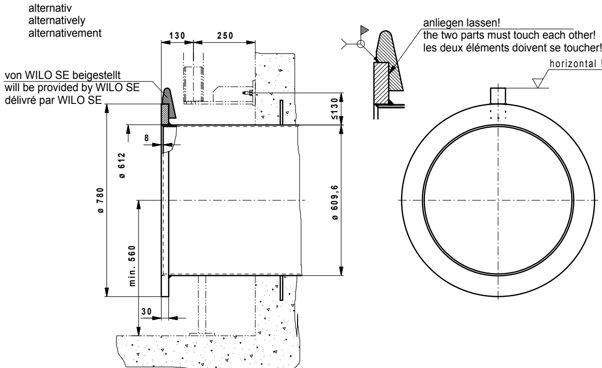
Druckrohr mit Stahling Discharge pipe with steel ring Tube de refoulement avec anneau en acier
