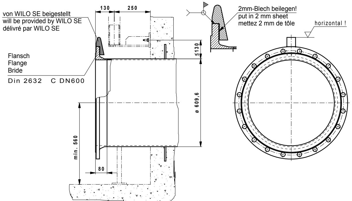
Druckrohr mit Vorschweißflansch Discharge pipe with welded flange Tube de refoulement avec bride soudée
