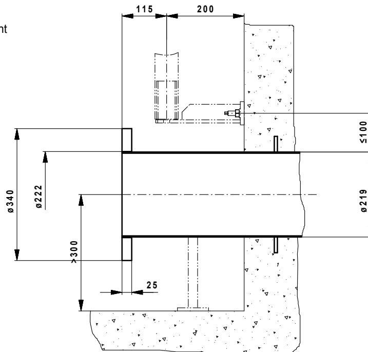
Druckrohr mit Stahling Discharge pipe with steel ring Tube de refoulement avec anneau en acier
