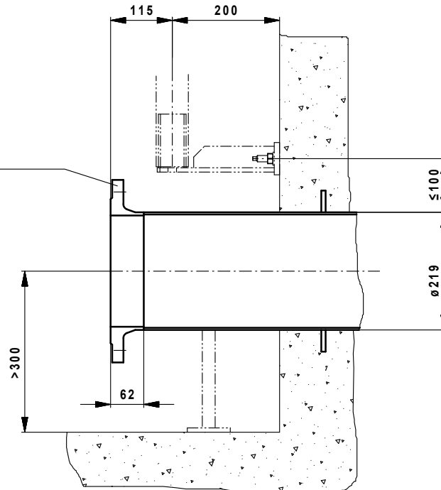
Druckrohr mit Vorschweißflansch Discharge pipe with welded flange Tube de refoulement avec bride soudée
