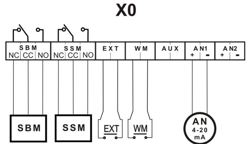
Рис. 3 Подсоединения сетевых контактов и клеммных колодок
