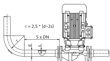
21. ábra: A szivattyú előtti és utáni csillapítási szakasz
