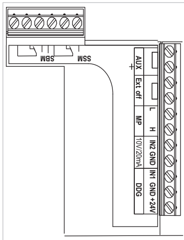
23. ábra: Vezérlőkapcsok
