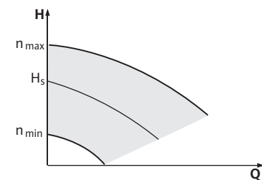
41. ábra: Állító üzemmód
