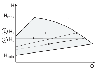
40. ábra: \Delta p -c/ \Delta p -v szabályozás
