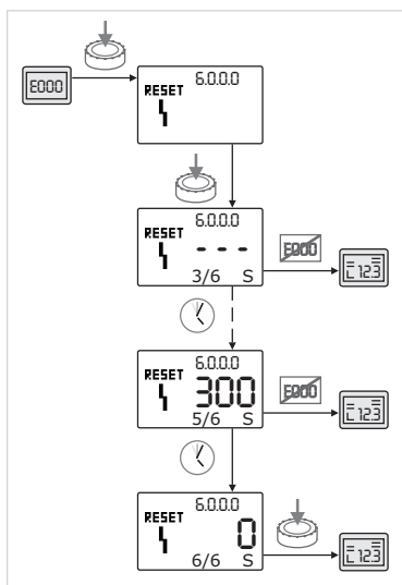
50. ábra: „C” hibatípus nyugtázása
