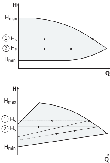
Σχ. 40: Τρόπος λειτουργίας Δρ-ε/Δρ-ν
