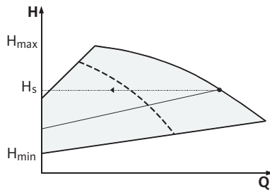
Σχ. 15: Ρύθμιση \Delta p-v (παράλληλη λειτουργία)
