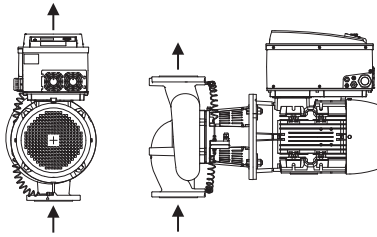
Fig. 17. Розташування компонентів у стані постачання
