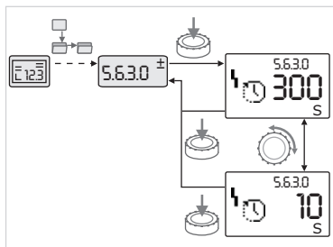
Fig. 37. Налаштування з поверненням до елемента меню «Вибір/налаштування»
