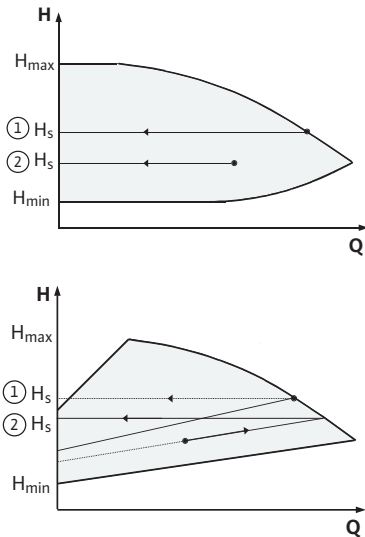
Fig. 42. Регулювання \Delta p -с/ \Delta p -v
