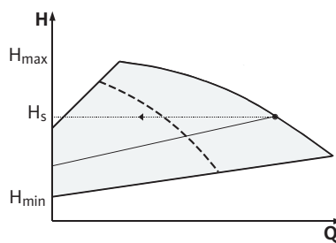
Fig. 15. Регулювання \Delta p -v (режим паралельної роботи)
