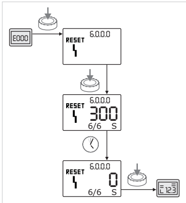
Fig. 50. Квитування помилок типу B (X = Y)
