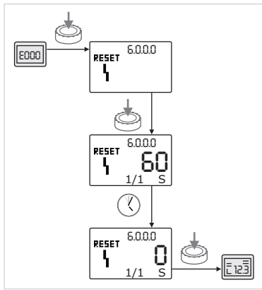
Fig. 47. Квитування помилок типу А або D
