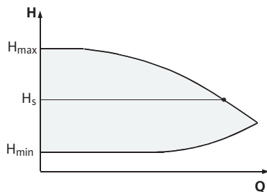
Fig. 10. Регулювання Др-с
