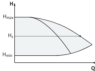
Fig. 14. Регулювання \Delta p -c (режим паралельної роботи)
