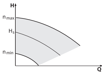
Fig. 43. Режим керування
