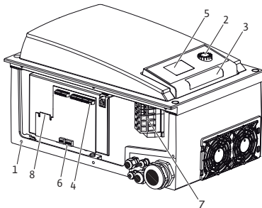
Fig. 9. Електронний модуль
