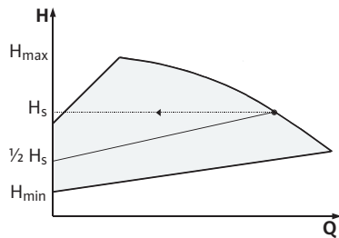
Fig. 11. Регулювання Др-ν
