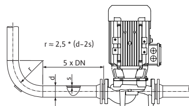
Fig. 21. Ділянка, на якій відбувається вирівнювання потоку, перед насосом та за ним
