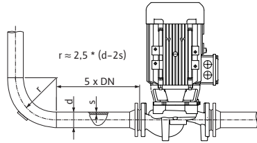
Fig. 21: Pompadan önceki ve pompadan sonraki sönümleme hattı
