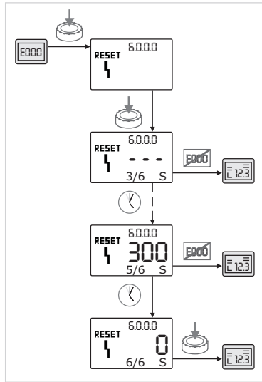
Fig. 52: Arıza tipi C'nin onaylanması
