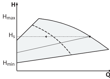
Fig. 15: Regülasyon \Delta p -v (paralel işletim)
