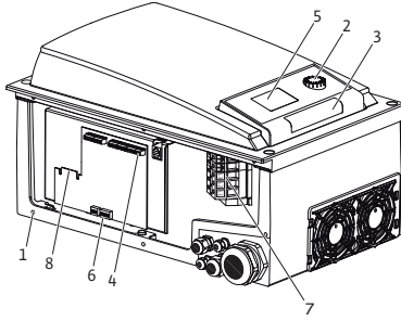
Fig. 9: Elektronik modül
