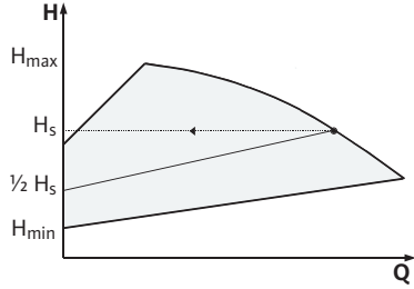
Fig. 11: Regülasyon \Delta p-v
