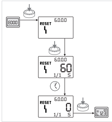
Fig. 47: Arıza tipi A veya D'nin onaylanması
