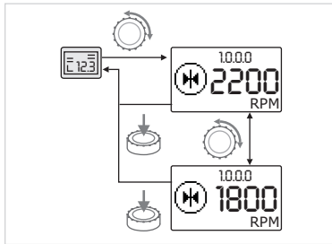
Fig. 32: Hedef değer girilmesi
