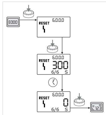
Fig. 50: Arıza tipi B'nin onaylanması (X=Y)
