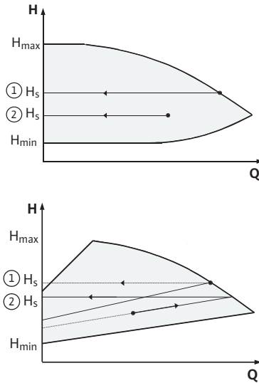
Fig. 42: Regülasyon \Delta p-c/\Delta p-v
