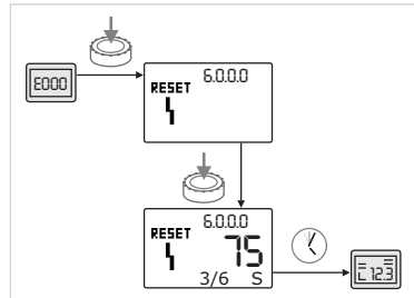
Fig. 49: Arıza tipi B'nin onaylanması (X < Y)
