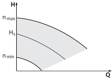
Fig. 12: Kontrol modu
