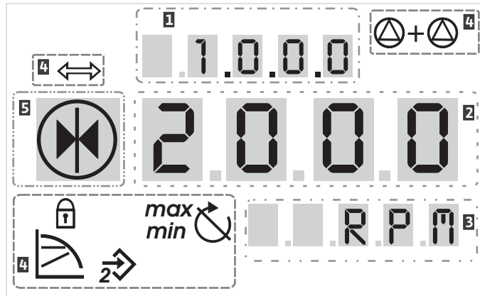
Fig. 29: Ekran yapısı
