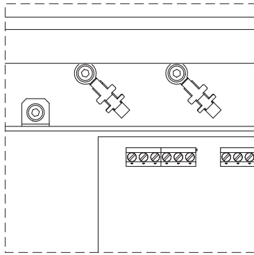
Fig. 23: Kablo zırhı
