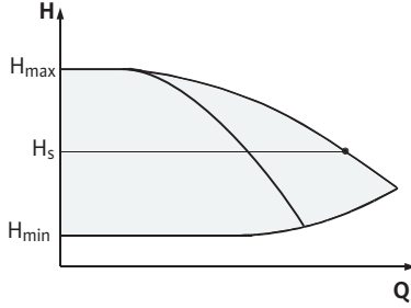
Fig. 14: Regülasyon \Delta p -c (paralel işletim)
