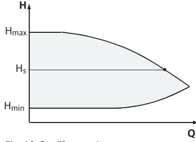
Fig. 10: Regülasyon \Delta p-c
