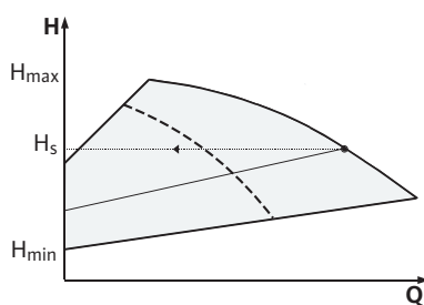
Fig. 15: Regulácia \Delta p -v (paralelný režim)
