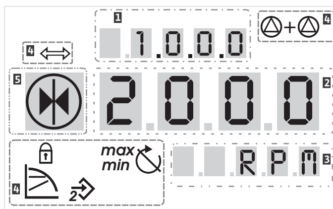
Fig. 29: Štruktúra displeja
