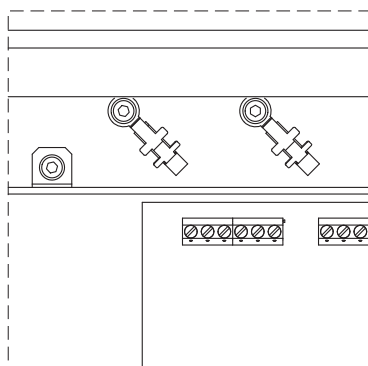
Fig. 23: Tienenie kábla
