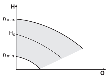
Fig. 12: Automatický režim s reguláciou otáčok
