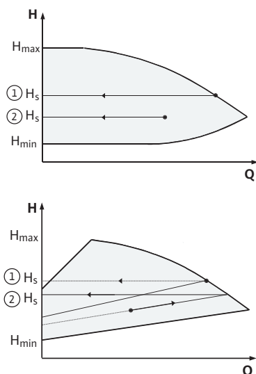
Fig. 42: Regulácia \Delta p\text{-c}/\Delta p\text{-v}
