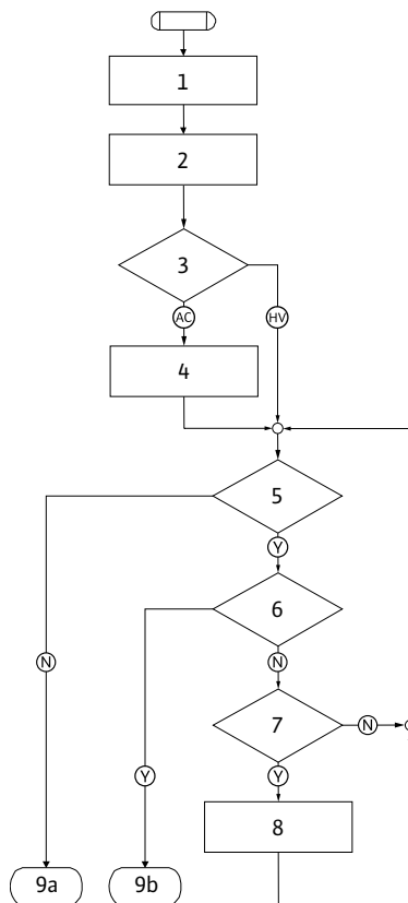
Fig. 53: E tipo klaidos, schema
