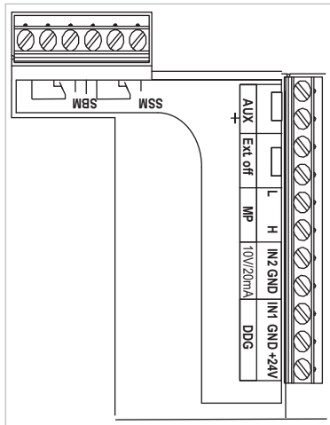
Fig. 24: Valdymo gnybtai
