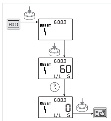
Fig. 47: A arba D tipo klaidos patvirtinimas
