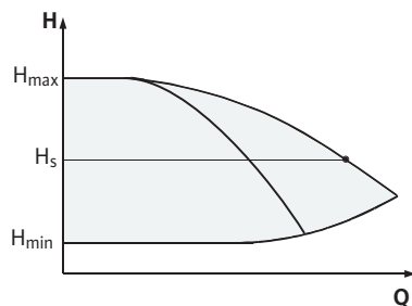
Fig. 14: Reguliavimas \Delta p -c (lygiagreto veikimo režimas)
