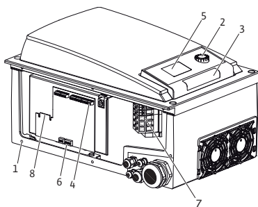
Fig. 9: Elektronikos modulis
