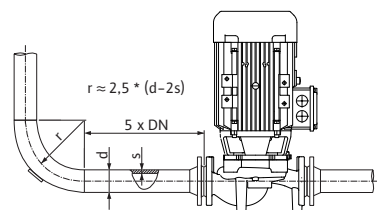
Fig. 21: Išlyginimo linija prieš siurblių ir už jo
