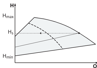
Fig. 15: Reguliavimas \Delta p -v (lygiagreto veikimo režimas)
