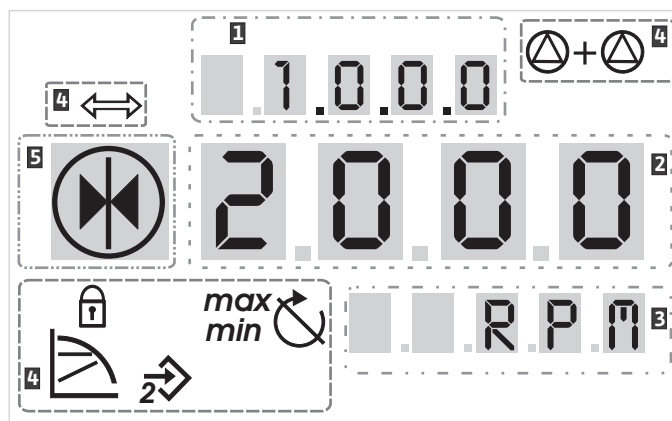
Fig. 29: Ekranų struktūra
