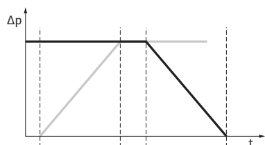
Fig. 16: Siurblių apsikeitimas
