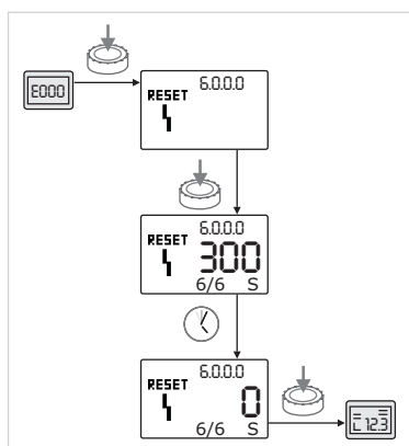
Fig. 50: B tipo klaidos patvirtinimas (X=Y)
