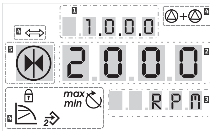
Fig. 29: A kijelző felépítése
