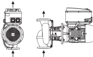
Fig. 17: Az alkatrészek elrendezése szállítási állapotban
