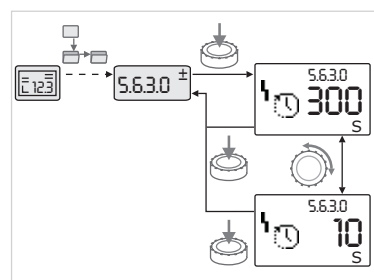
Fig. 37: Beállítás a „kiválasztás/beállítások” menüelemhez történő visszatéréssel
