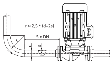
Fig. 21: A szivattyú előtti és utáni csillapítási szakasz
