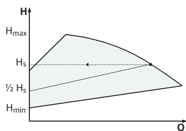
Fig. 11: \Delta p -v szabályzás
