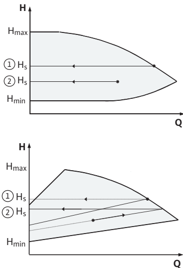
Fig. 42: \Delta p -c/ \Delta p -v szabályzás
