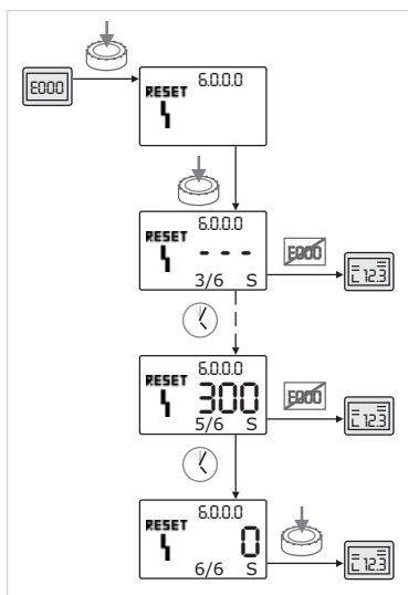
Fig. 52: „C” hibatípus nyugtázása
