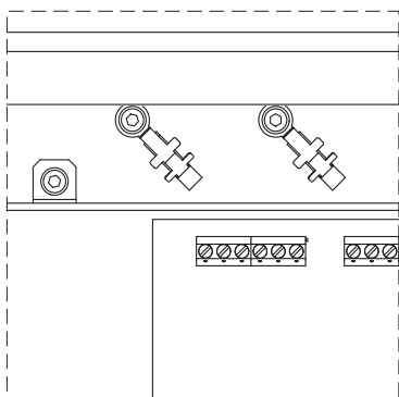
Fig. 23: Kábelárnyékolás
