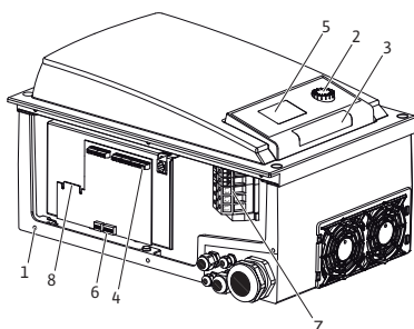
Fig. 9: Elektronikamodul
