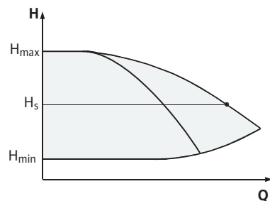
Fig. 14: \Delta p -c szabályzás (párhuzamos üzem)
