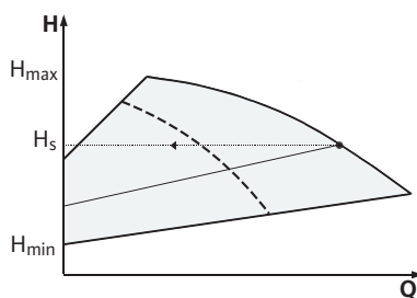
Fig. 15: \Delta p -v szabályzás (párhuzamos üzem)
