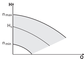
Fig. 43: Állító üzemmód
