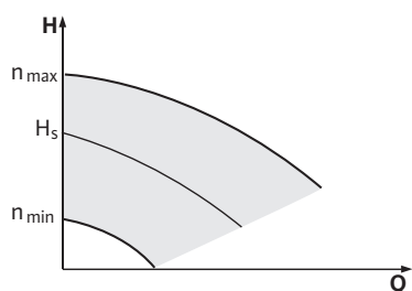
Fig. 12: Állító üzemmód
