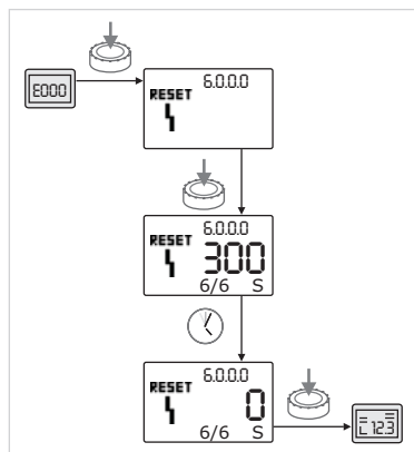
Fig. 50: „B” hibatípus nyugtázása ( X = Y )
