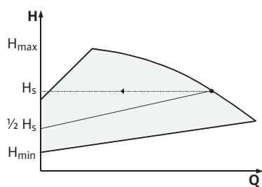
Fig. 11: Регулиране Δp-v
