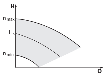
Fig. 43: Режим на управление
