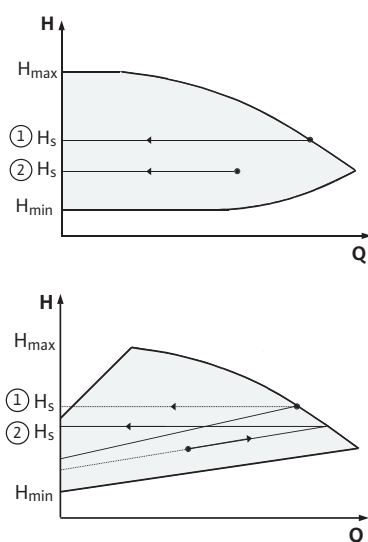
Fig. 42: Регулиране \Delta p-s/\Delta p-v
