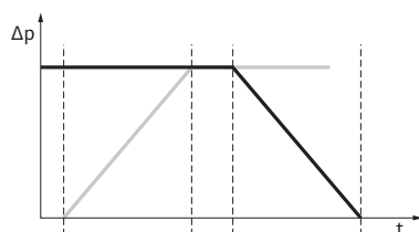
Fig. 16: Размяна на помпите
