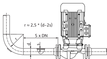
Fig. 21: Успокоителна отсечка преди и след помпата
