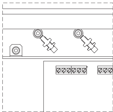
Fig. 23: Екраниране на кабелите
