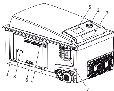
Fig. 9: Електронен модул
