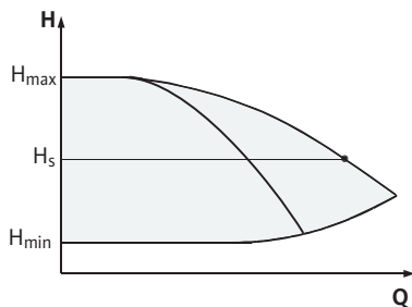
Fig. 14: Регулиране Др-с (паралелна работа)
