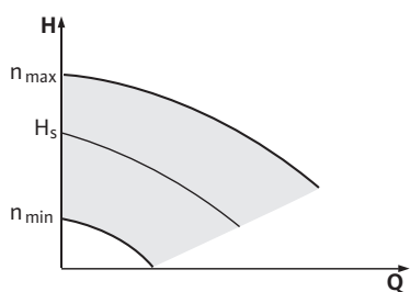
Fig. 12: Режим на управление
