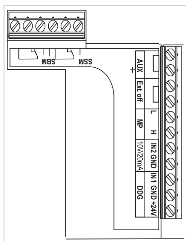
Fig. 24: Управляващи клеми
