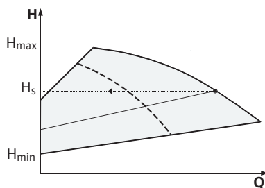
Fig. 15: Регулиране Др-в (паралелна работа)
