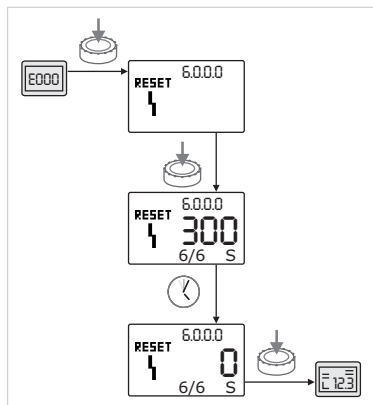
Fig. 50: Зачистване на грешки от тип В ( X=Y )
