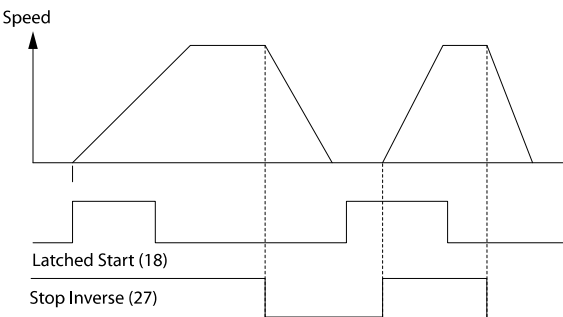
Bild 6.3 Pulsstart-/stopp, inverterat
