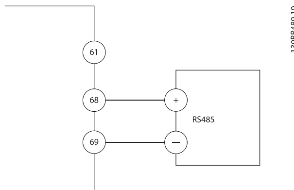
Bild 4.28 Kopplingsschema för seriell kommunikation
