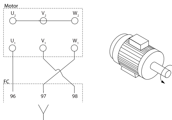
Bild 5.5 Kabeldragning för att ändra motorriktning
