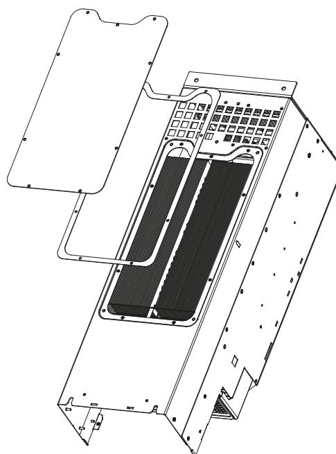
Bild 7.1 Åtkomstpanel för kylplatta
