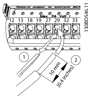
Bild 4.26 Ansluta styrkablar
