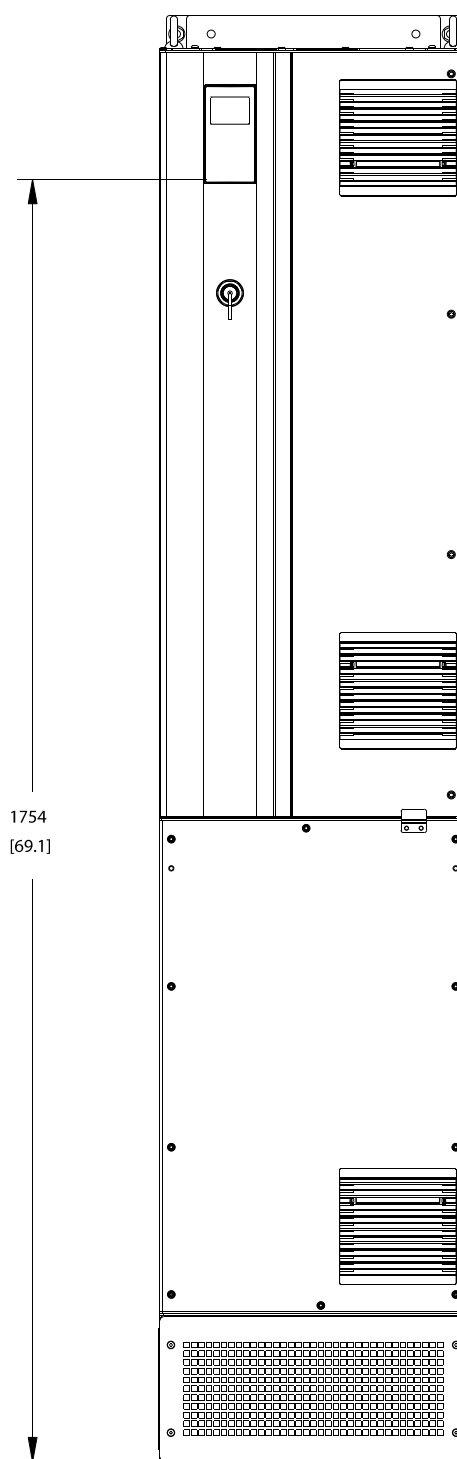
Slika 1.2 Kućište D7h
