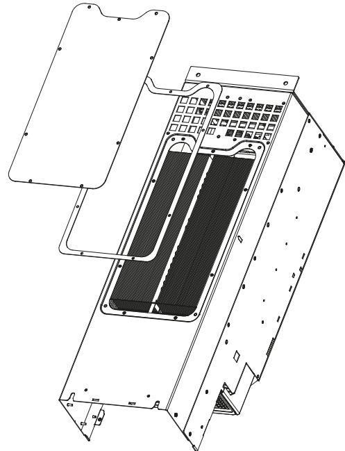
Slika 7.1 Panel za pristup hladnjaku
