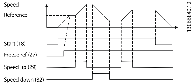
Slika 6.1 Povećanje/smanjenje brzine
