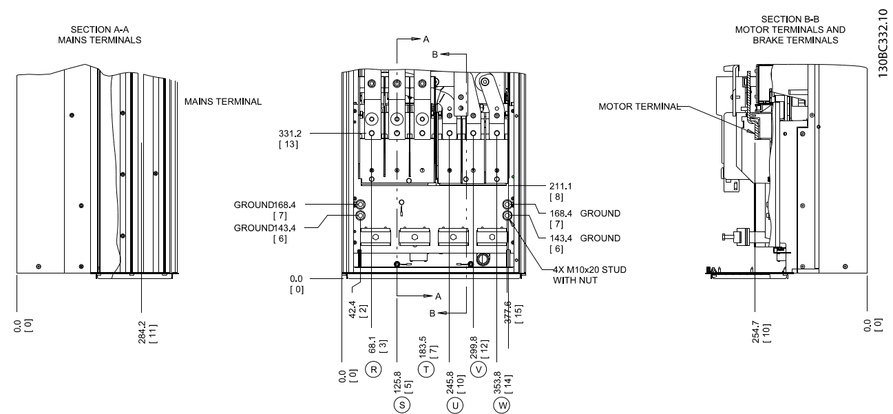
Slika 4.6 Lokacije priključka, D2h
