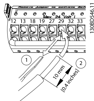
Afbeelding 4.26 Stuurkabels aansluiten
