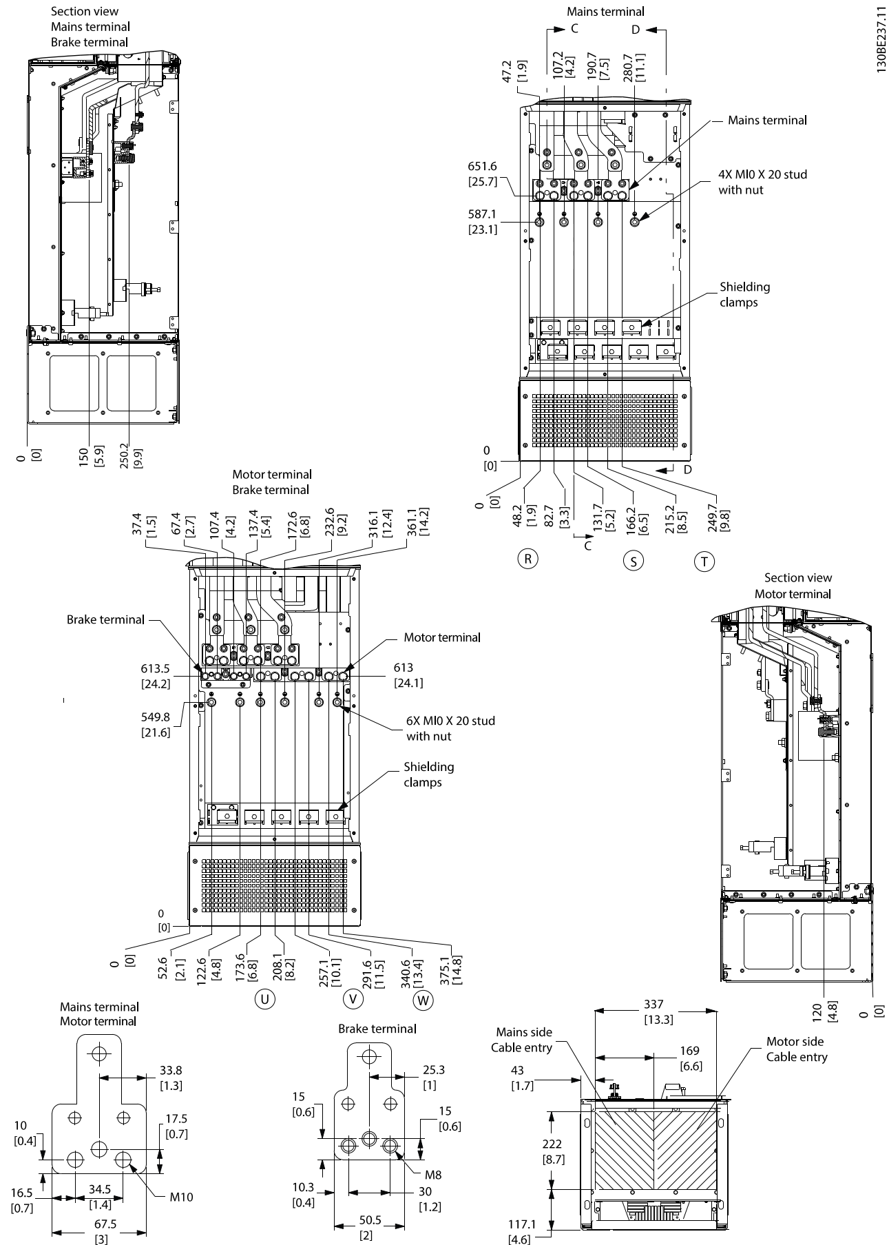
Afbeelding 4.19 Overgedimensioneerde kabelkast, D7h
