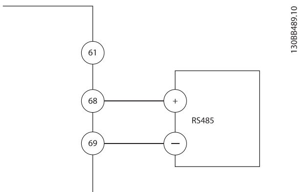
Afbeelding 4.28 Bedradingsschema voor seriële communicatie
