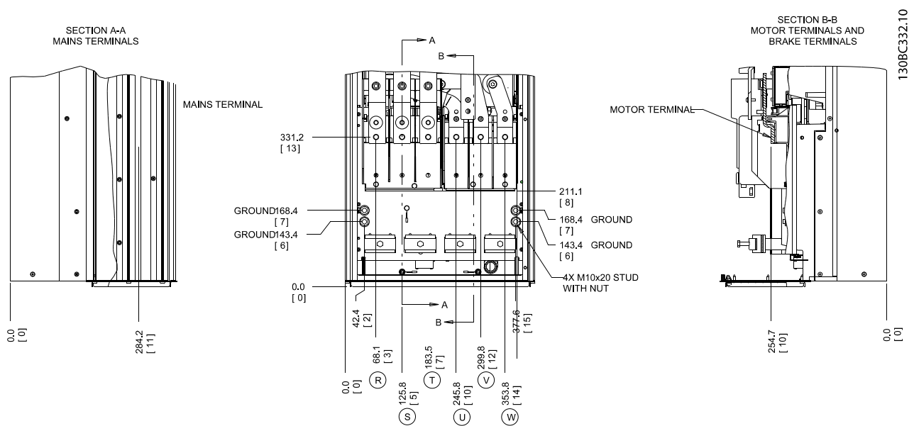
Afbeelding 4.6 Klemposities, D2h
