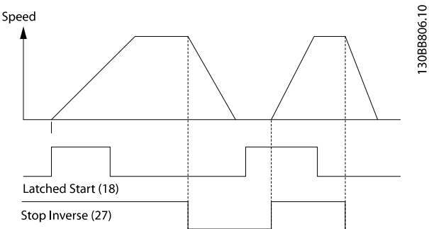
Afbeelding 6.3 Pulsstart/Stop geïnverteerd
