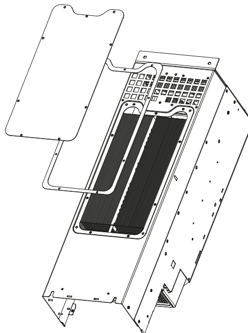
Afbeelding 7.1 Toegangspaneel koellichaam
