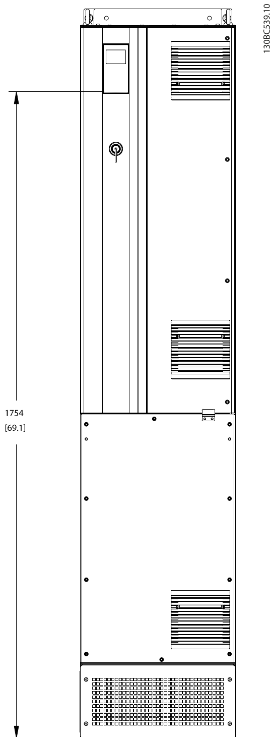
Afbeelding 1.2 D7h-behuizing
