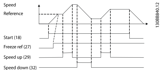
Afbeelding 6.1 Snelheid omhoog/omlaag
