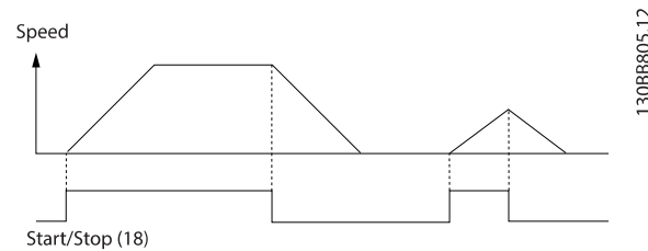
Afbeelding 6.2 Start-/stopcommando met STO
