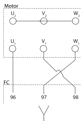
Afbeelding 5.5 Bedrading voor wijziging van de draairichting van de motor
