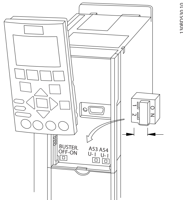
Afbeelding 4.27 Positie van de schakelaars voor klem 53 en 54
