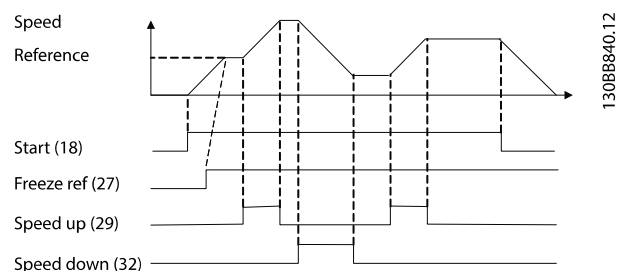
Ábra 6.1 Fordulatszám-növelés és -csökkentés
