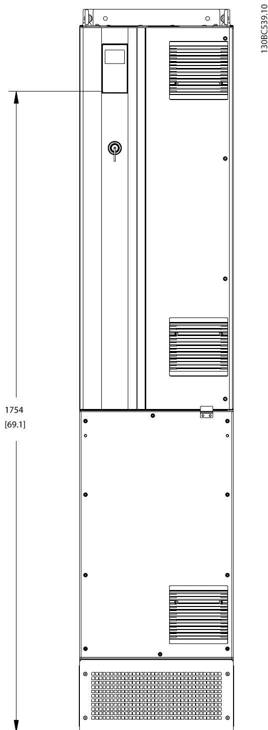
Ábra 1.2 D7h ház méret
