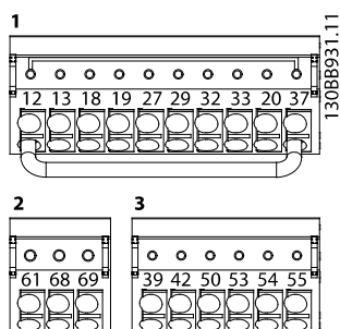
Ilustración 4.25 Números de los terminales
