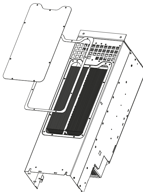
Ilustración 7.1 Panel de acceso a disipador
