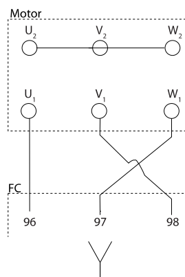
Illustration 5.5 Ledningsføring for ændring af motorretning
