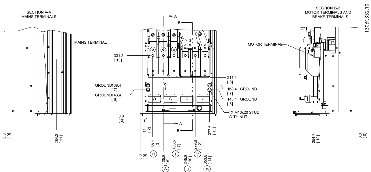
Illustration 4.6 Klemmeplaceringer, D2h
