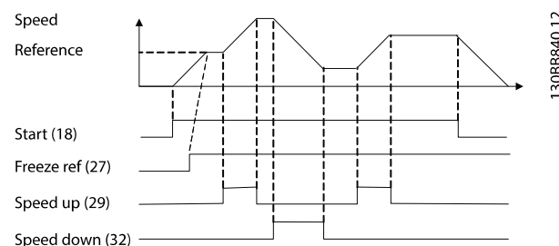
Illustration 6.1 Hastighed op/ned
