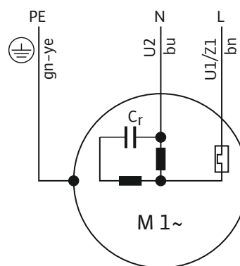
Fig. 7: Plán pripojenia 1~–motora
