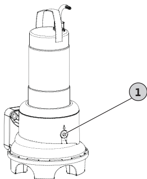
Fig. 10: Tesniaca komora: Výmena oleja
