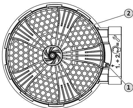
Fig. 9: Odmontovanie základovej dosky
