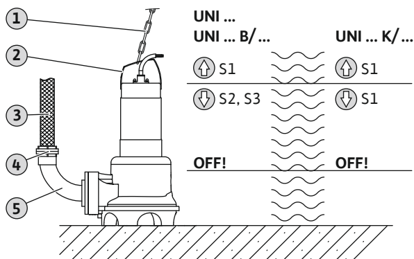
Fig. 6: Inštalácia do mokrého prostredia, mobilná
