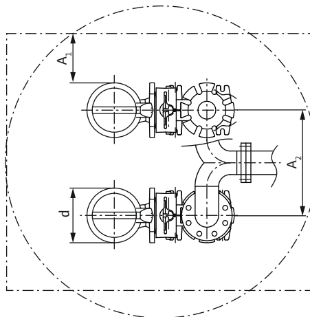
Fig. 3: Minimálne vzdialenosti
