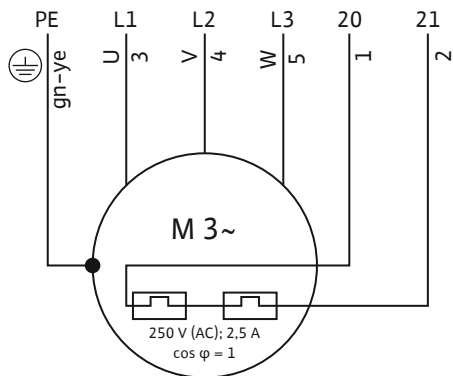
Fig. 8: Plán pripojenia 3~motora
