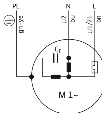
Fig. 7: Anslutningsschema 1~motor
