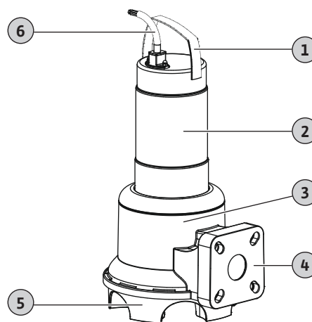
Fig. 2: Översikt
