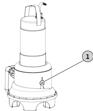
Fig. 10: Tätningkammare: Oljebyte
