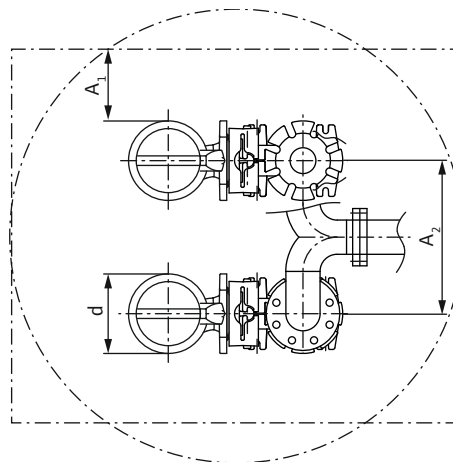
Fig. 3: Minsta avstånd
