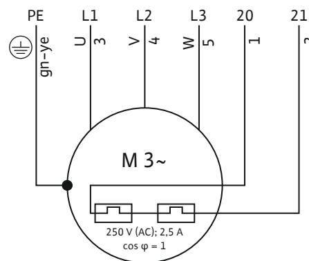
Fig. 8: Anslutningsschema 3~motor
