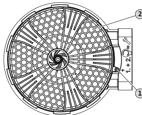
Fig. 9: Demontera bottenplattan
