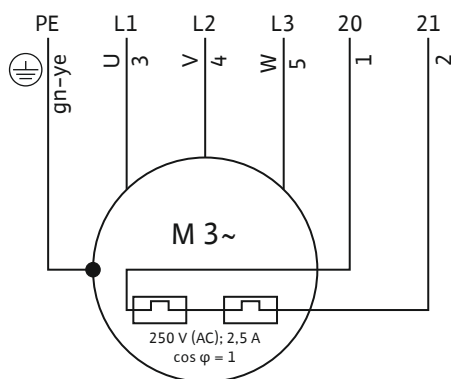
Fig. 8: Σχεδιάγραμμα σύνδεσης 3~ κινητήρας
