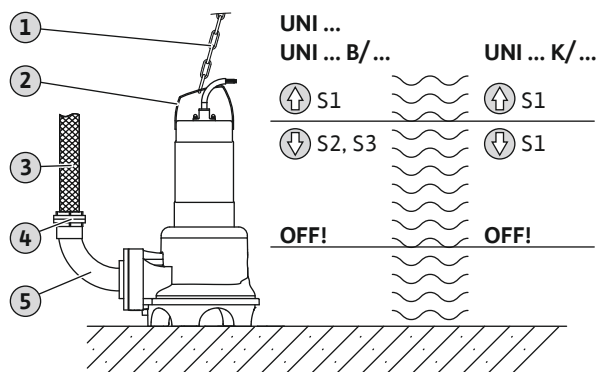
Fig. 6: Υγρή εγκατάσταση εντός φρεατίου, φορητή
