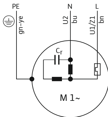
Fig. 7: Σχεδιάγραμμα σύνδεσης 1~ κινητήρας
