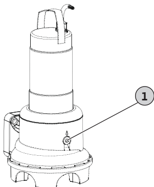
Fig. 10: Θάλαμος στεγανοποίησης: Αλλαγή λαδιού
