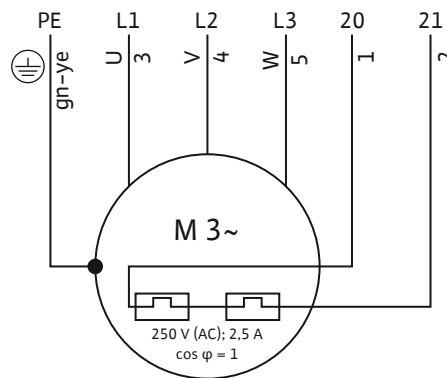
Fig. 8: Tilslutningsdiagram 3~motor
