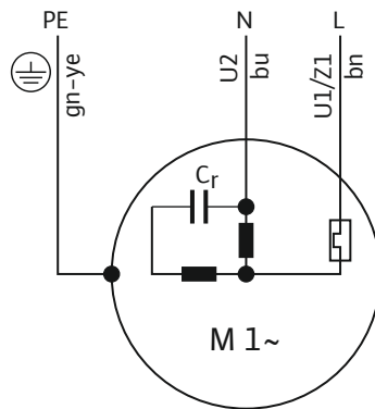
Fig. 7: Tilslutningsdiagram 1~motor
