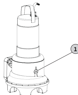
Fig. 10: Tætningskammer: Olieskift
