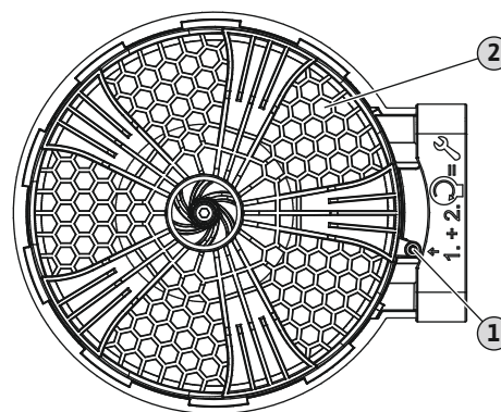
Fig. 9: Afmontering af bundplade
