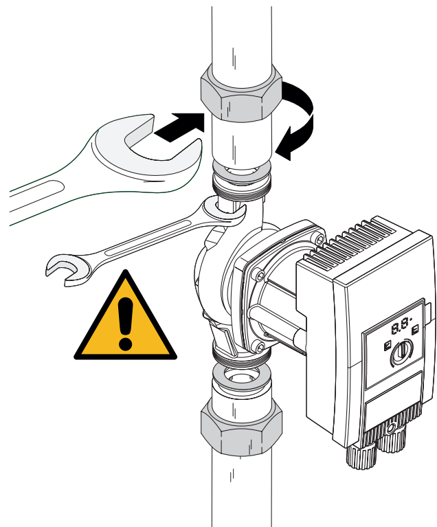
Fig. 11: Монтиране на помпа
