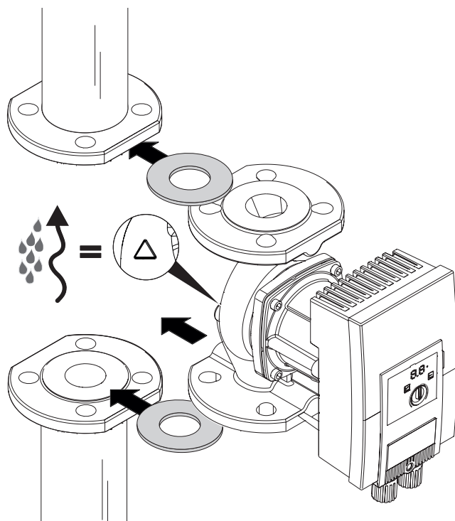
Fig. 7: Монтиране на помпата
