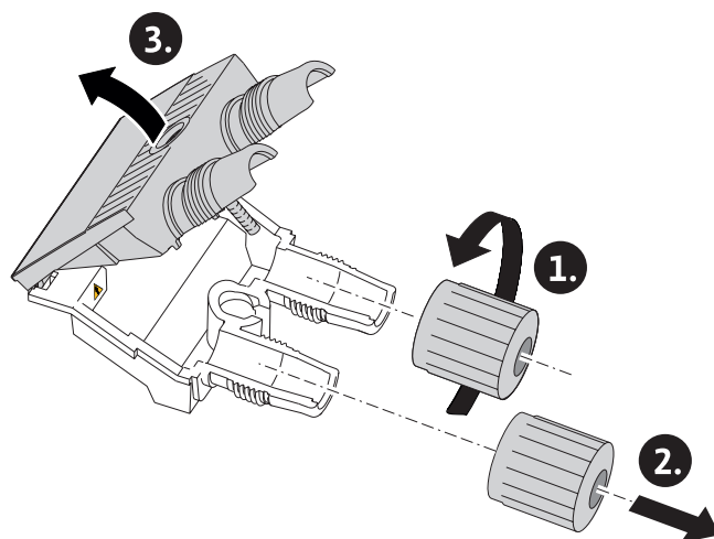
Fig. 17: Отваряне на щепсел
