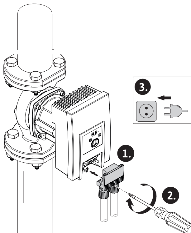
Fig. 21: Монтиране на щепсел
