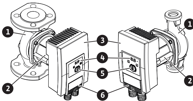
Fig. 1: Преглед на помпи с фланцово и резбово тръбно присъединяване (единична помпа)
