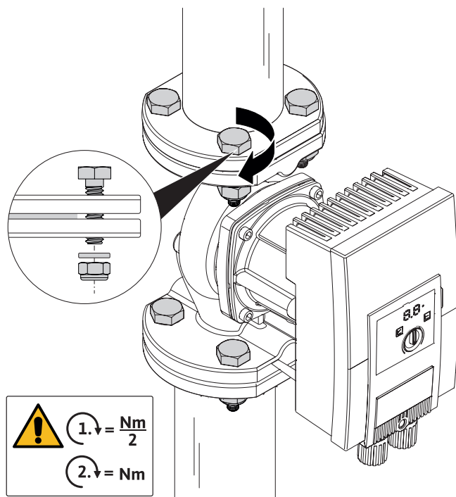
Fig. 8: Монтиране на помпа
