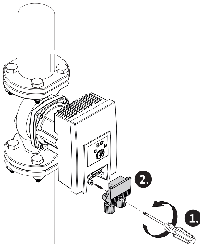
Fig. 16: Демонтиране на щепсел
