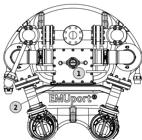
Fig. 23: Nettoyage de l'aspiration et de la conduite de trop-plein
