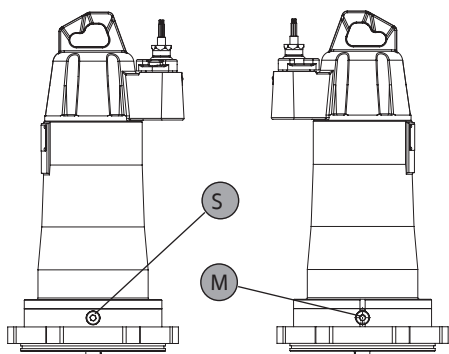
Fig. 26: Moteur FK 17.1
