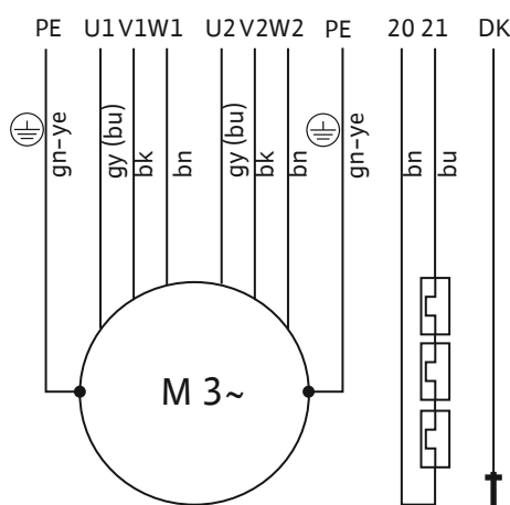
Fig. 15: Schéma de raccordement : FK 202, démarrage étoile-triangle, sonde PTO, avec câble de raccordement NSSHÖU-J à 2x 4 fils et câble de contrôle
