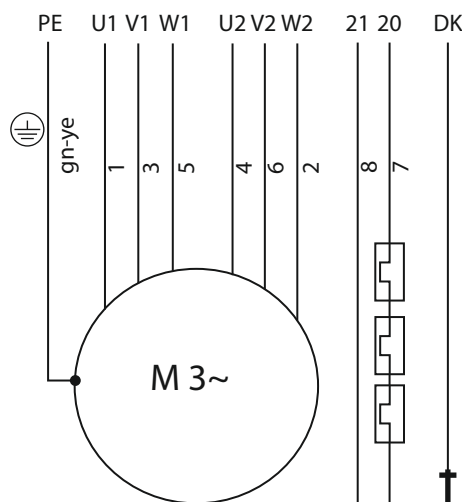
Fig. 13: Schéma de raccordement : FK 17.1, démarrage étoile-triangle, sonde PTO, avec câble de raccordement H07RN-F à 10 fils
