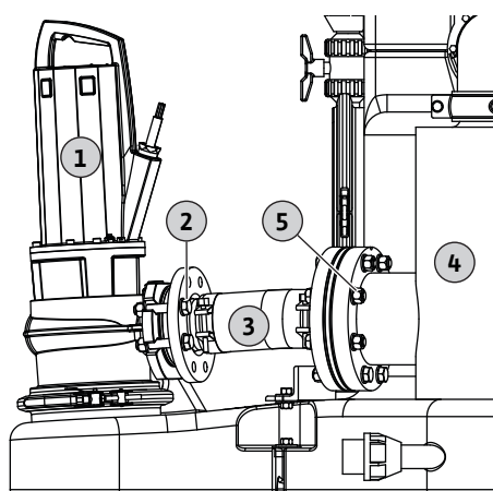
Fig. 24: Nettoyage des cuves de séparation des solides
