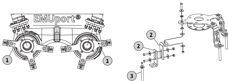
Fig. 8: Supports de fixation de la pompe
