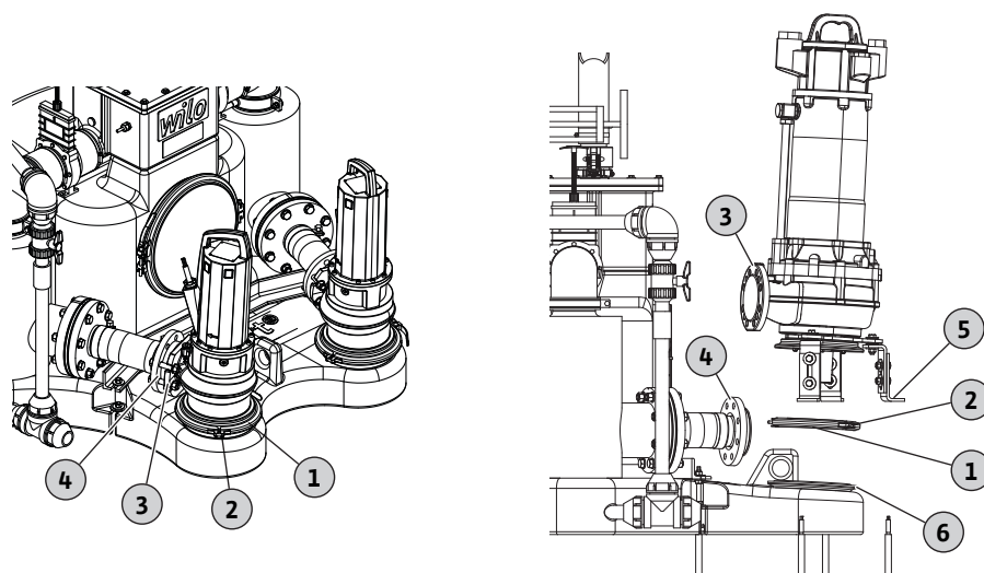
Fig. 7: Installation des pompes pour eaux chargées
