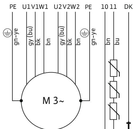
Fig. 16: Schéma de raccordement : FK 202, démarrage étoile-triangle, capteur PTC, avec câble de raccordement NSSHÖU-J à 2x 4 fils et câble de contrôle
