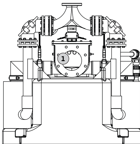
Fig. 5: Raccordement de l'aspiration
