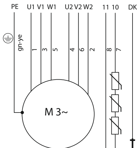
Fig. 14: Schéma de raccordement : FK 17.1, démarrage étoile-triangle, capteur PTC, avec câble de raccordement H07RN-F à 10 fils
