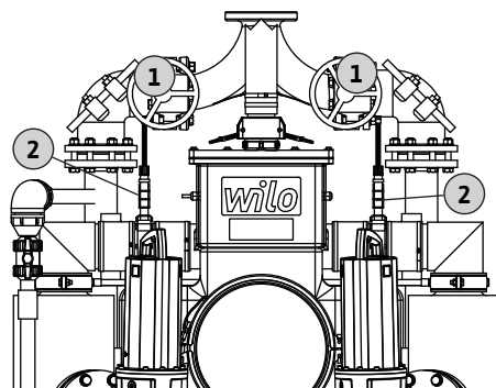
Fig. 21: Aperçu des vannes d'arrêt
