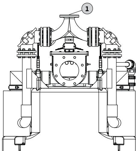
Fig. 4: Raccordement du raccord de refoulement
