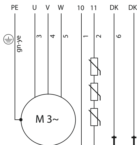
Fig. 10: Schéma de raccordement : P 13, démarrage direct, capteur PTC, avec câble de raccordement H07RN-F ou TGSH à 7 fils
