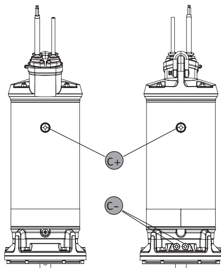
Fig. 29: Moteur FKT 20.2
