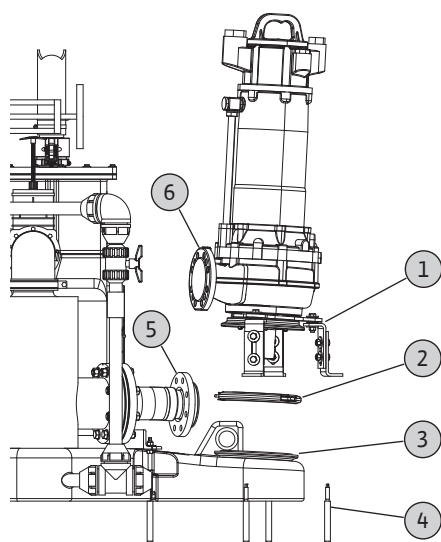
Fig. 30: Retrait des pompes pour eaux chargées
