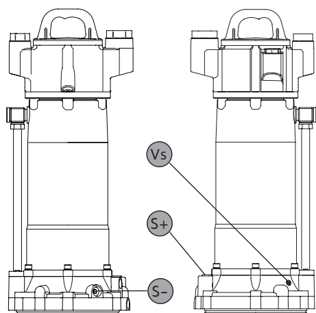
Fig. 28: Vidange d'huile de la chambre d'étanchéité FK 202
