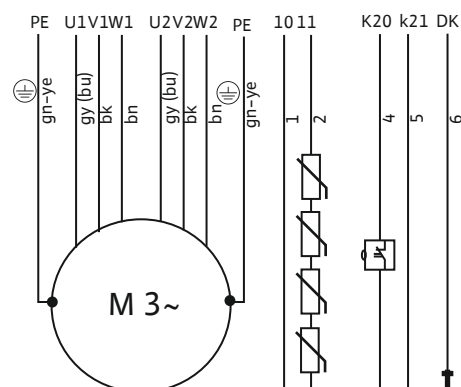
Fig. 19: Schéma de raccordement : FKT 20.2, démarrage étoile-triangle, capteur PTC, avec câble de raccordement NSSHÖU-J à 2x 4 fils et câble de contrôle
