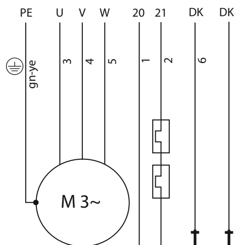
Fig. 9: Schéma de raccordement : P 13, démarrage direct, sonde PTO, avec câble de raccordement H07RN-F ou TGSH à 7 fils
