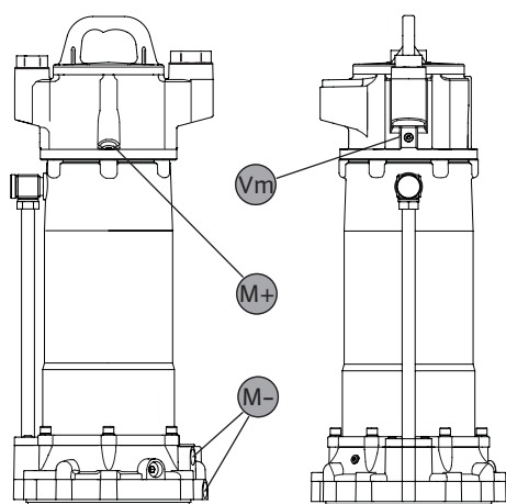
Fig. 27: Vidange d'huile du compartiment moteur FK 202
