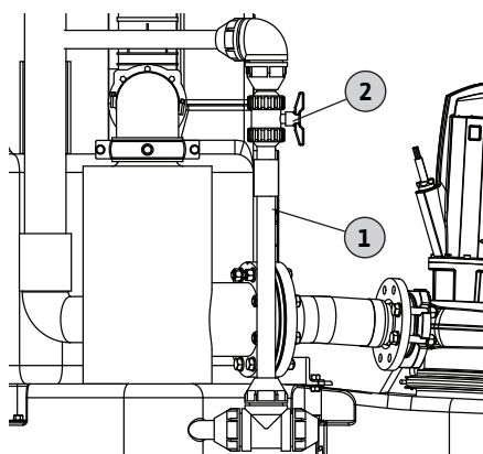
Fig. 20: Conduite de rinçage du réservoir collecteur
