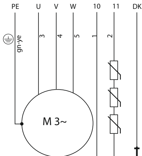
Fig. 12: Schéma de raccordement : FK 17.1, démarrage direct, capteur PTC, avec câble de raccordement H07RN-F à 7 fils
