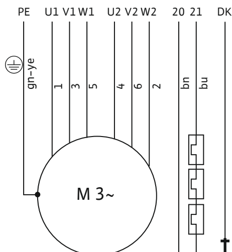
Fig. 17: Schéma de raccordement : FK 202, démarrage étoile-triangle, sonde PTO, avec câble de raccordement H07RN-F à 7 fils et câble de contrôle
