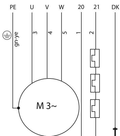
Fig. 11: Schéma de raccordement : FK 17.1, démarrage direct, sonde PTO
