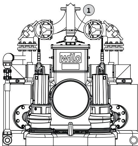
Fig. 6: Raccord de purge du réservoir collecteur
