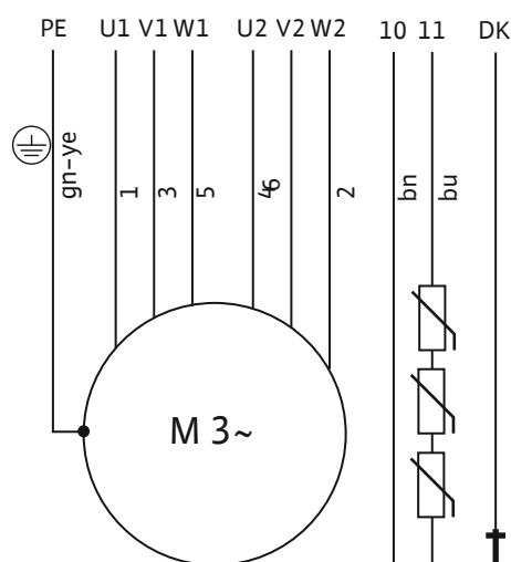
Fig. 18: Schéma de raccordement : FK 202, démarrage étoile-triangle, capteur PTC, avec câble de raccordement H07RN-F à 7 fils et câble de contrôle
