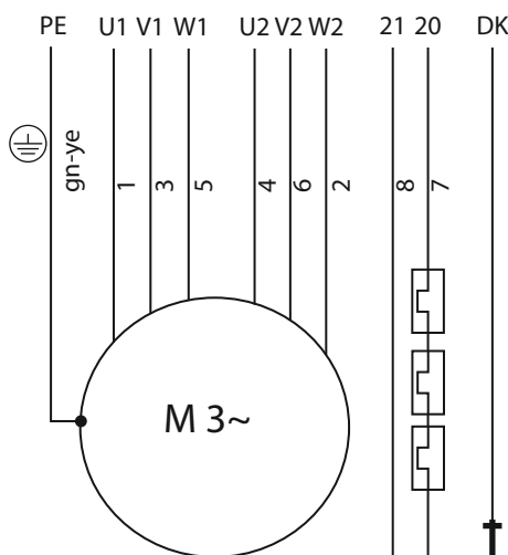
Fig. 13: Anschlussplan: FK 17.1, Stern-Dreieck-Schaltung, Bimetallfühler, mit 10-adrigem H07RN-F-Anschlusskabel
