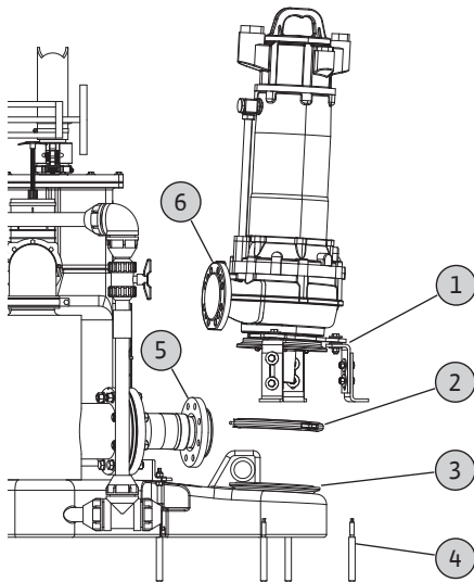
Fig. 30: Abwasserpumpen ausbauen
