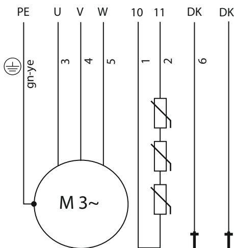
Fig. 10: Anschlussplan: P 13, Direktanlauf, PTC-Fühler, mit 7-adrigem H07RN-F- oder TGSH-Anschlusskabel
