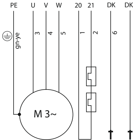
Fig. 9: Anschlussplan: P 13, Direktanlauf, Bimetallfühler, mit 7-adrigem H07RN-F- oder TGSH-Anschlusskabel
