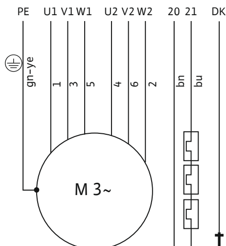
Fig. 17: Anschlussplan: FK 202, Stern-Dreieck-Schaltung, Bimetallfühler, mit 7-adrigem H07RN-F-Anschlusskabel und Steuerkabel
