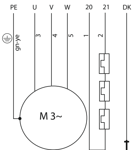
Fig. 11: Anschlussplan: FK 17.1, Direktanlauf, Bimetallfühler
