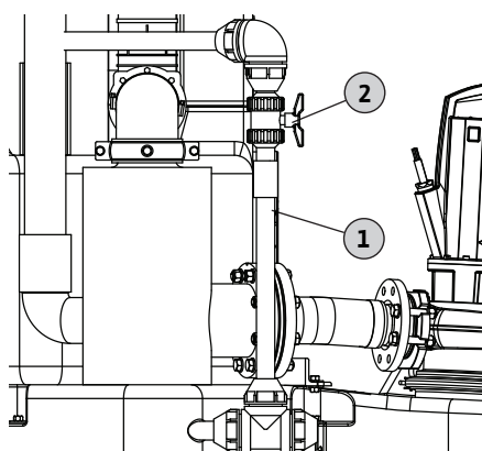
Fig. 20: Leitung zum Spülen des Sammelbehälters
