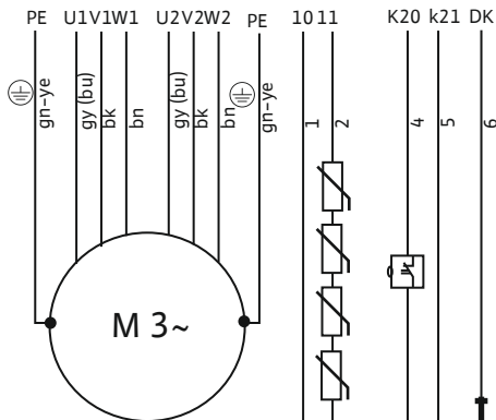
Fig. 19: Anschlussplan: FKT 20.2, Stern-Dreieck-Schaltung, PTC-Fühler, mit 2x 4-adrigem NSSHÖU-J-Anschlusskabel und Steuerkabel
