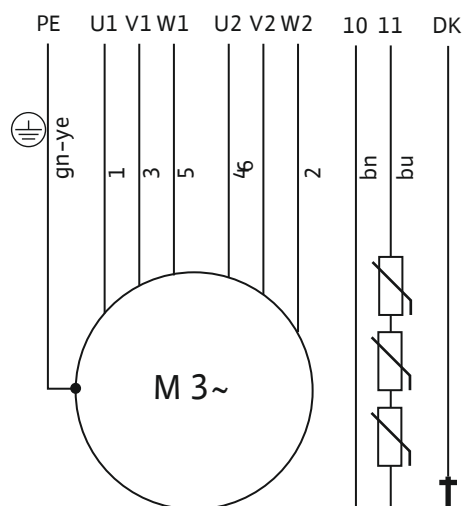
Fig. 18: Anschlussplan: FK 202, Stern-Dreieck-Schaltung, PTC-Fühler, mit 7-adrigem H07RN-F-Anschlusskabel und Steuerkabel
