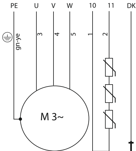
Fig. 12: Anschlussplan: FK 17.1, Direktanlauf, PTC-Fühler, mit 7-adrigem H07RN-F-Anschlusskabel
