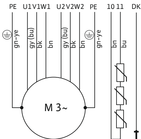
Fig. 16: Anschlussplan: FK 202, Stern-Dreieck-Schaltung, PTC-Fühler, mit 2x 4-adrigem NSSHÖU-J-Anschlusskabel und Steuerkabel
