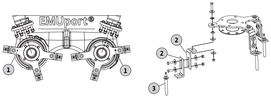
Fig. 8: Pumpenhalterungen
