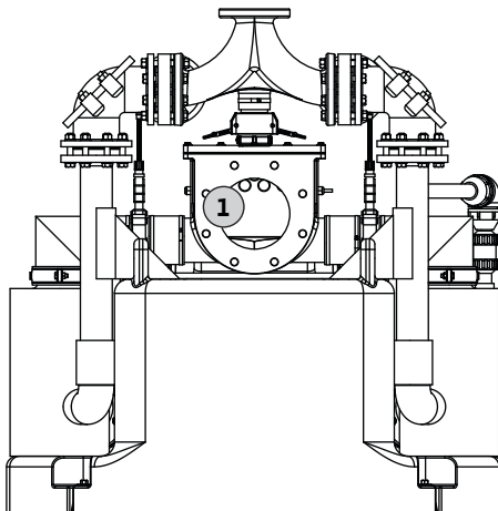
Fig. 5: Zulauf anschließen
