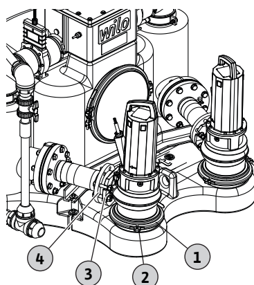
Fig. 7: Die Abwasserpumpen aufstellen
