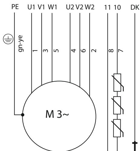
Fig. 14: Anschlussplan: FK 17.1, Stern-Dreieck-Schaltung, PTC-Fühler, mit 10-adrigem H07RN-F-Anschlusskabel
