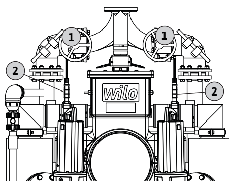
Fig. 21: Übersicht der Absperrarmaturen
