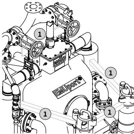
Fig. 2: Transportsicherung
