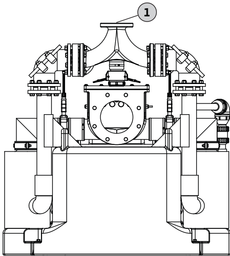
Fig. 4: Druckanschluss anbringen
