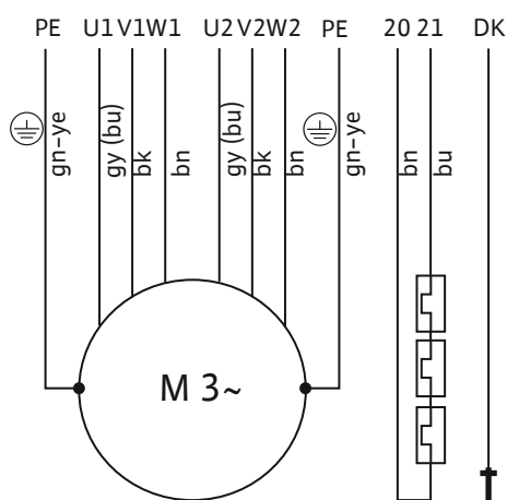
Fig. 15: Anschlussplan: FK 202, Stern-Dreieck-Schaltung, Bimetallfühler, mit 2x 4-adrigem NSSHÖU-J-Anschlusskabel und Steuerkabel
