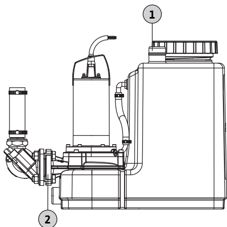
Fig. 6: Під'єднання для видалення повітря збірний резервуар
