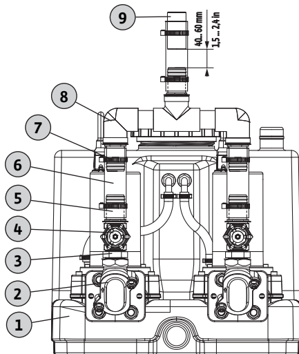
Fig. 3: Установка напірного патрубку
