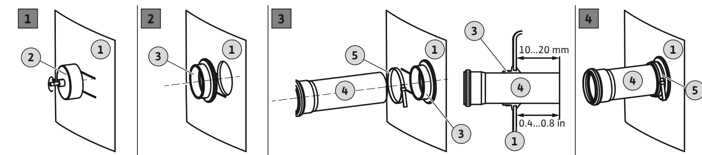
Fig. 5: Připojení přítoku
