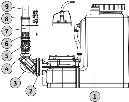
Fig. 3: Установка напірного патрубку
