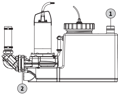
Fig. 8: Під'єднання для видалення повітря збірного резервуара
