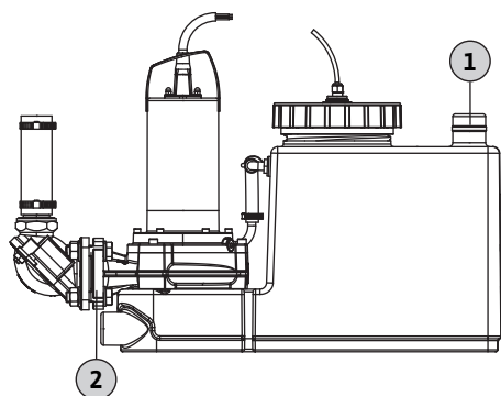
Fig. 8: Priključak za ventilaciju sabirnog rezervoara
