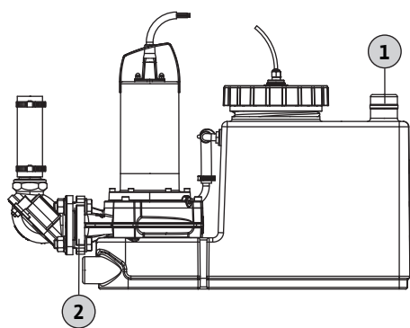
Fig. 8: Racordul de dezaerisire al recipientului colector
