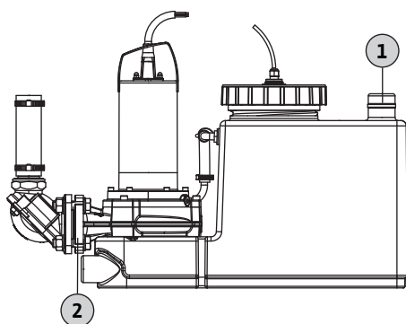
Fig. 8: Przyłącze odpowietrzające zbiornika retencyjnego
