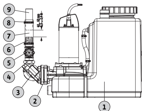
Fig. 3: Montaż przyłącza tłocznego
