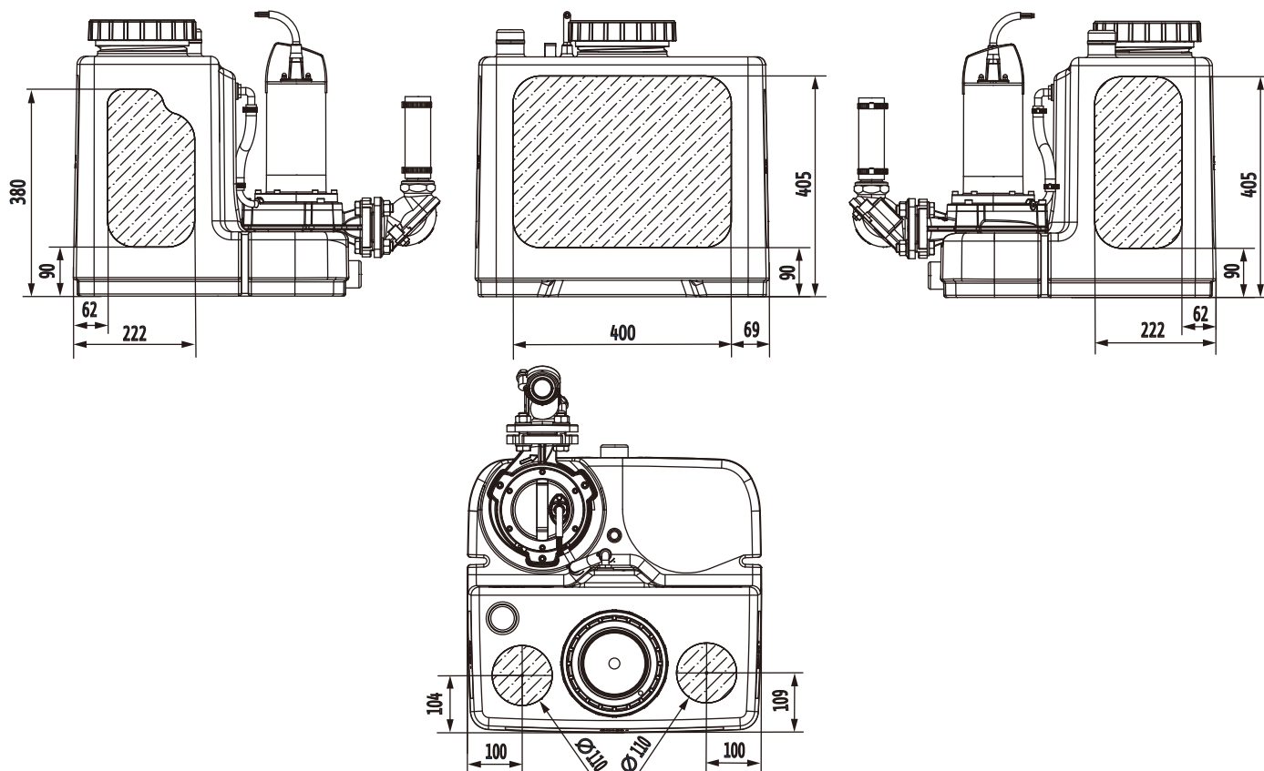
Fig. 4: Innløpsområder
