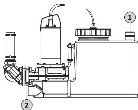
Fig. 8: Raccordo di aerazione e del serbatoio di raccolta
