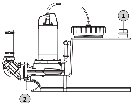
Fig. 8: Priključak za odzračivanje sabirnog spremnika
