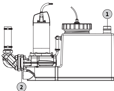
Fig. 8: Keräyssäiliön ilmanpoistoliitäntä
