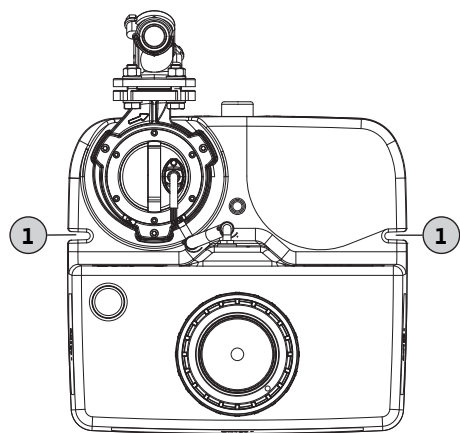
Fig. 2: Näkymä pumppaamosta ylhäältäpäin
