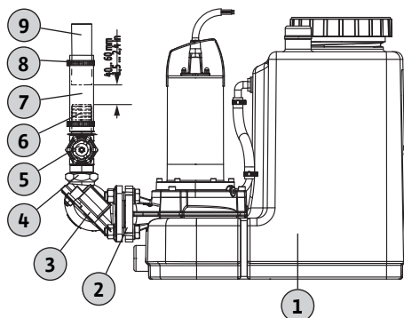
Fig. 3: Paineliitännän asennus
