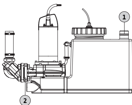
Fig. 8: Conexión de purga del depósito colector
