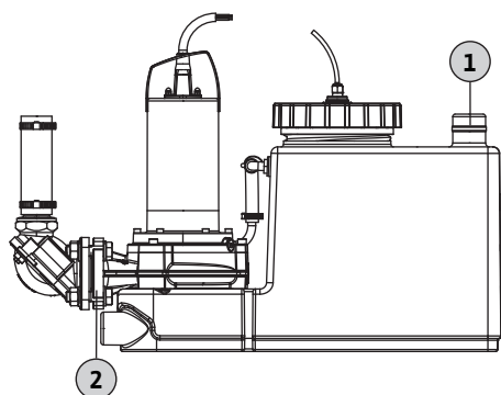
Fig. 8: Σύνδεση εξαερισμού δεξαμενής συλλογής λυμάτων
