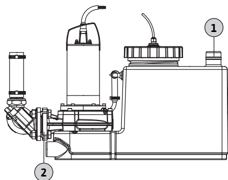
Fig. 8: Извод за обезвъздушаване на събирателния резервоар
