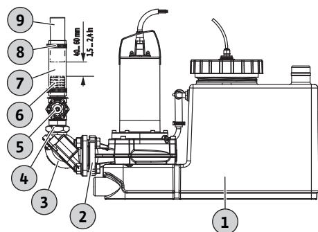
Fig. 3: Postavljanje potisnog priključka
