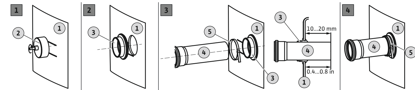
Fig. 5: Подсоединение приточного отверстия
