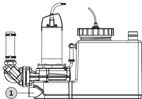
Fig. 6: Verbinding van de handmembraanpomp
