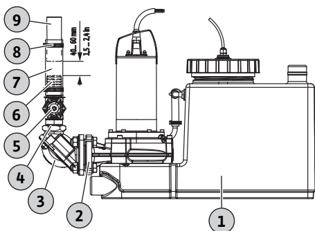
Fig. 3: Paineliitännän asennus
