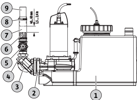
Fig. 3: Montaje de la conexión de impulsión
