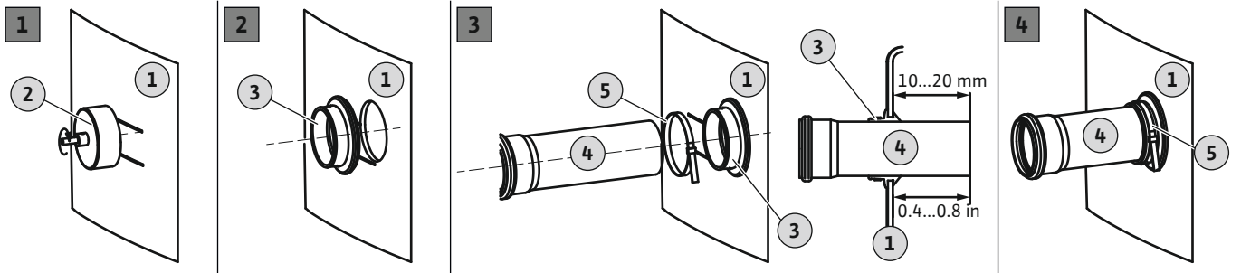
Fig. 5: Girişi bağlama
