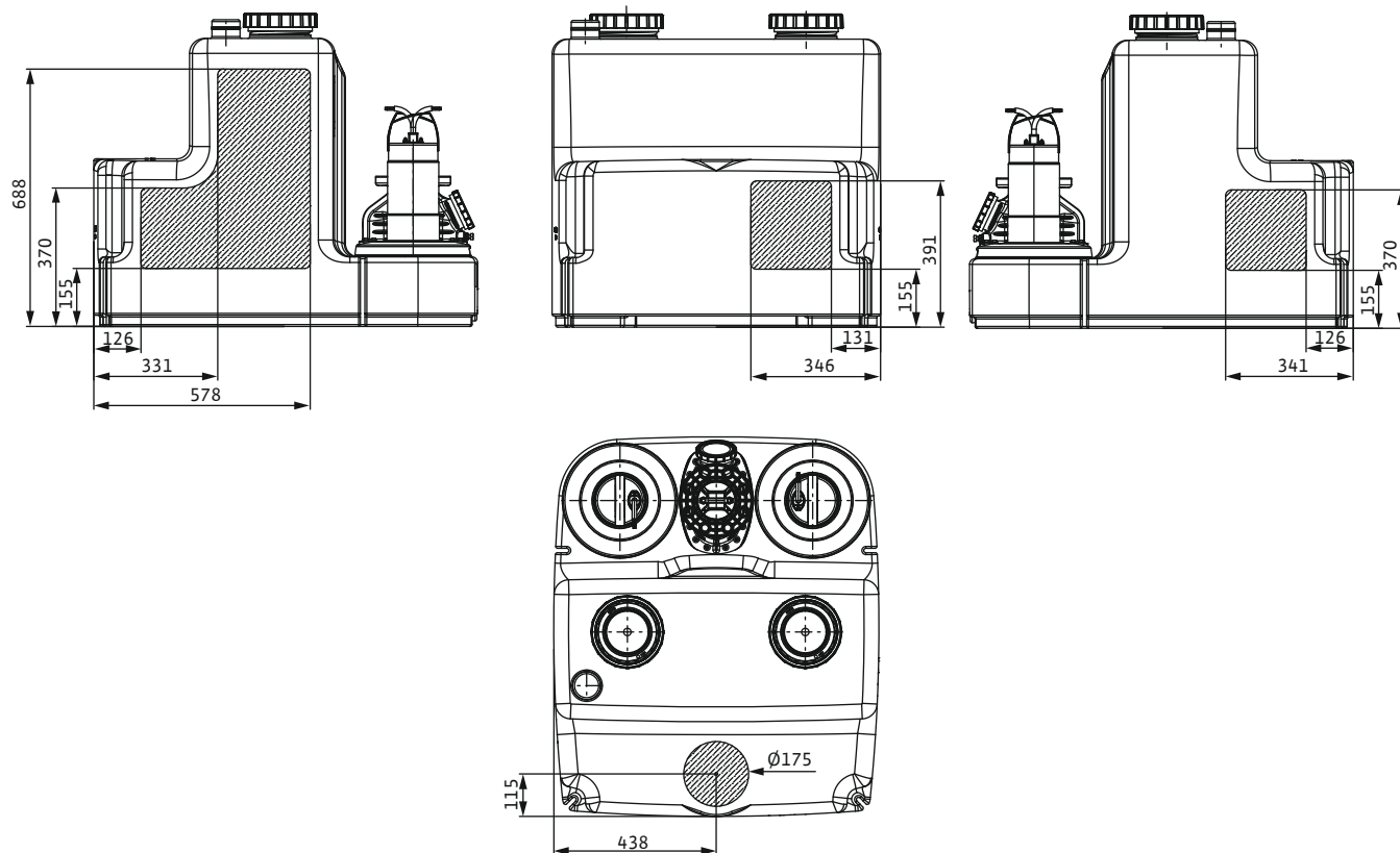
Fig. 4: Innløpsområder
