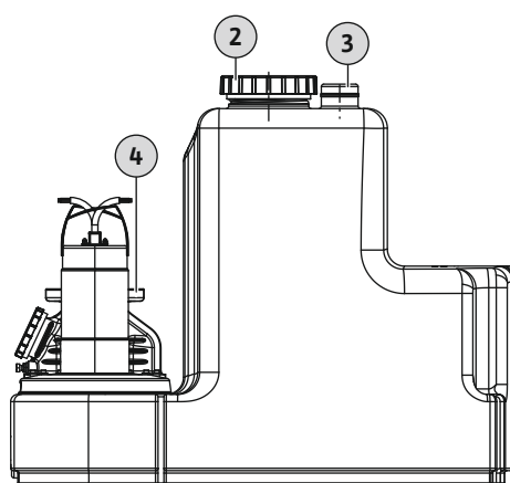
Fig. 6: Raccord de purge du réservoir collecteur
