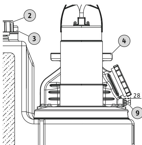
Fig. 8: Ilmaustulpan aseointi
