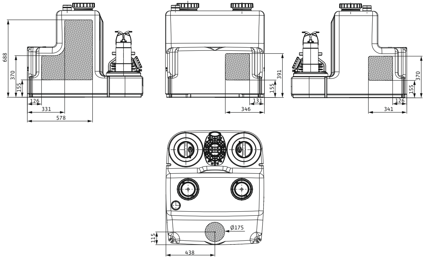
Fig. 4: Tulovirtausalueet
