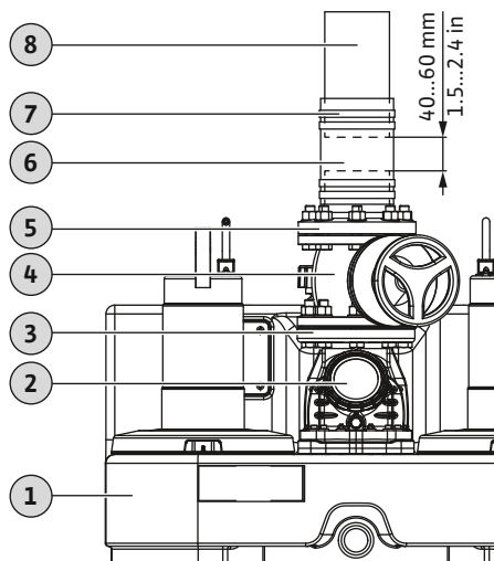
Fig. 3: Paineliitännän asennus
