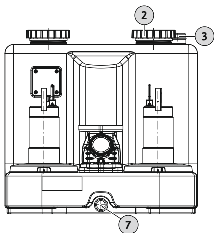
Fig. 7: Свързване на ръчна мембранна помпа
