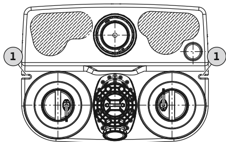
Fig. 2: Gornji pregled uređaja za odvođenje otpadnih voda
