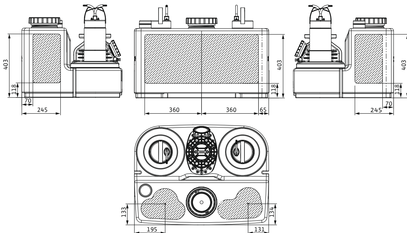
Fig. 4: Obszary dopływu
