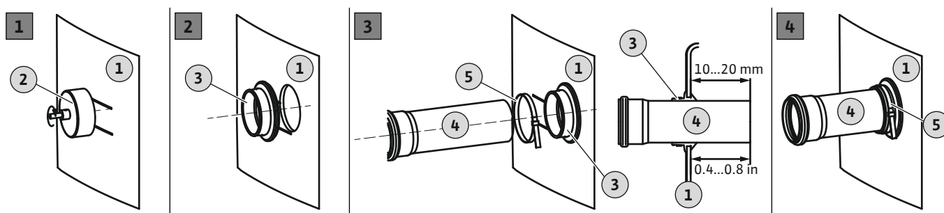
Fig. 5: Podłączenie dopływu
